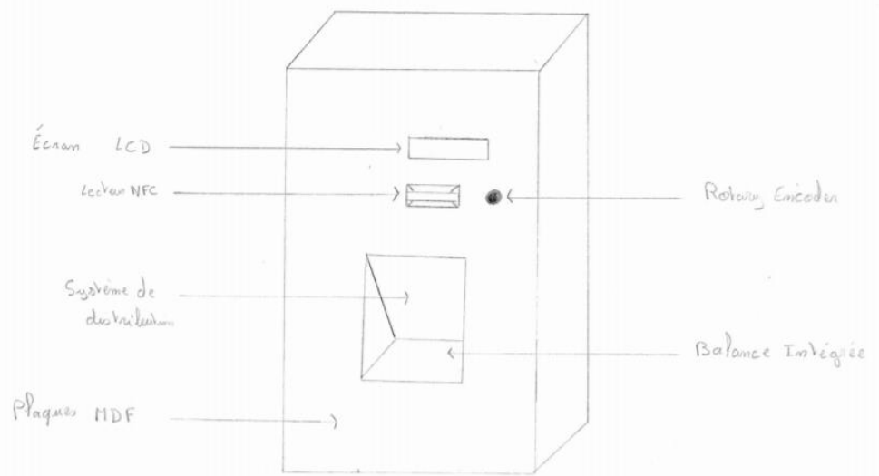
Schéma du Distributeur [ Vue de Face ]
