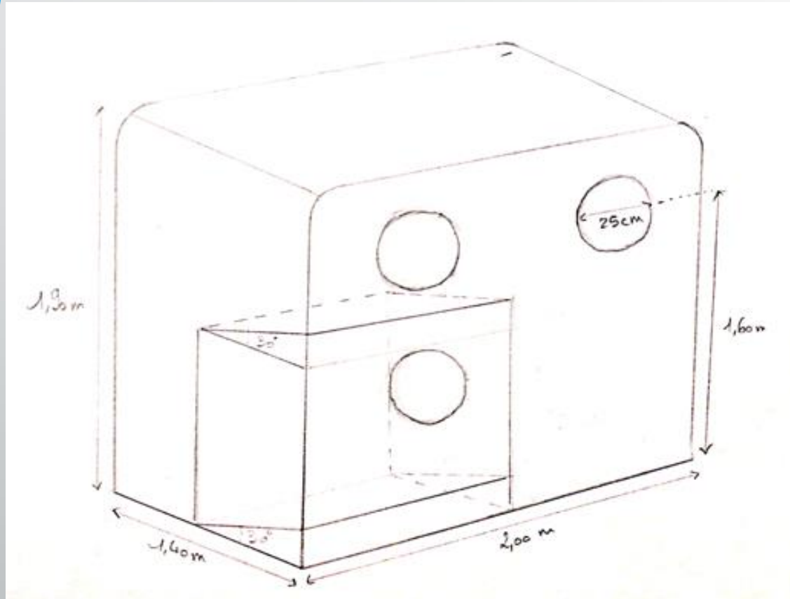
Schéma du projet fini
